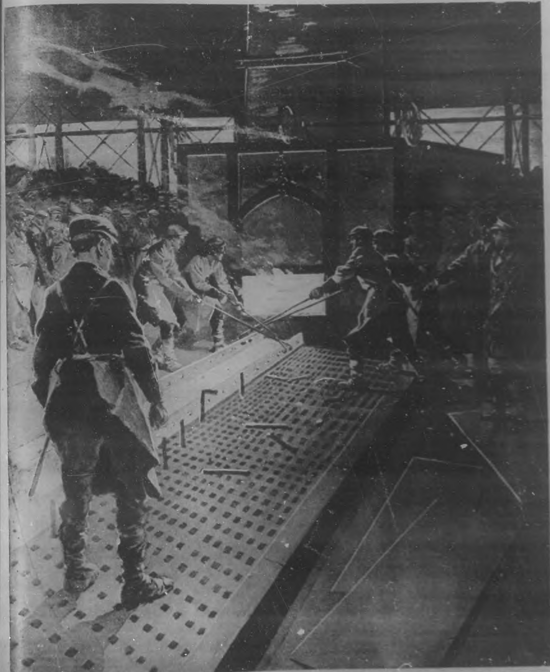
El Príncipe de Gales ( a la derecha, en primer término) presenciando los trabajos de fundición de piezas de acero con destino a los grandes acorazados que construye Inglaterra en sus talleres navales.
